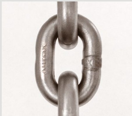
Hebezeugketten QHK hohe Maßgenauigkeit/enge Toleranzen Größe 7,0 x 21,0 mm
